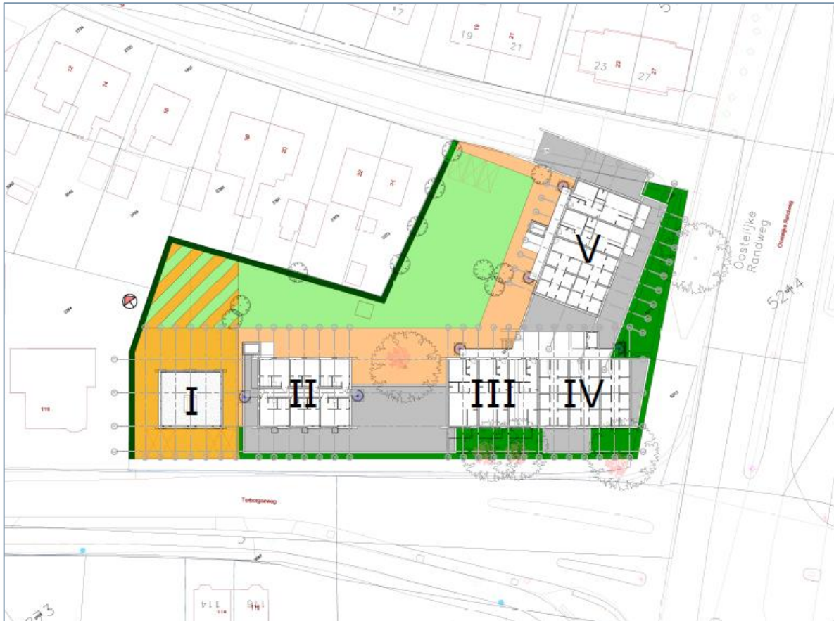
Figuur 2. Structuurontwerp Appartements Terborgseweg. Bron: WBC Bouwgroep (29 juni 2021, gewijzigd: 18-03-2022 en 11-07-2022).
